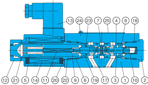
03 SNH-G04-AR-**-10 06
