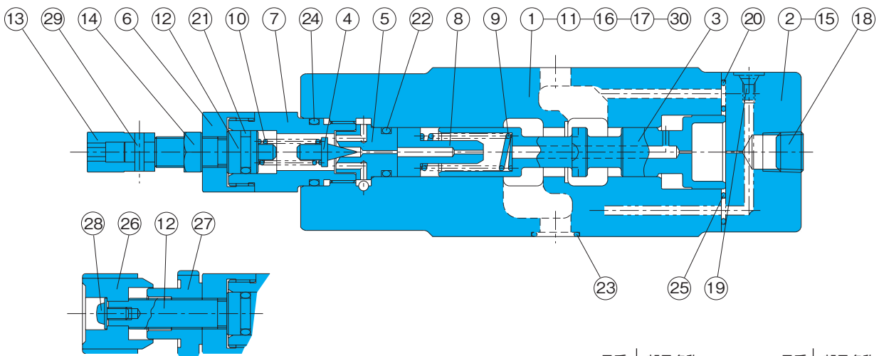
シール部品一覧表 (キット形式 BRES-O3GC*-1A)
